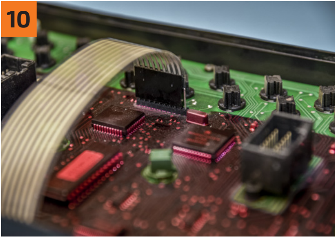
Verbinden Sie das Flachbandkabel mit den Steckkontakten auf der Platine. ACHTUNG: Ein Pin bleibt frei. Achten Sie unbedingt auf die Ausrichtung der Pins und des Flachbandkabels.
